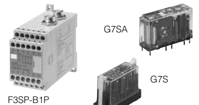
F3SP-B1P
